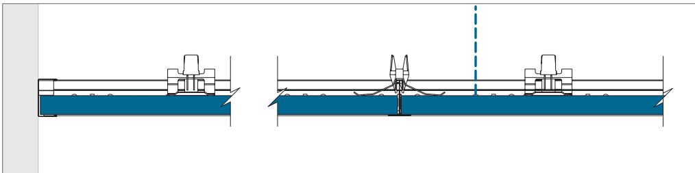
Wykończenia przyściennie z profilem C i ze sprężyną przyścienną dociskową dla płyty o grubości 20 mm (odporność na uderzenia 3A).
